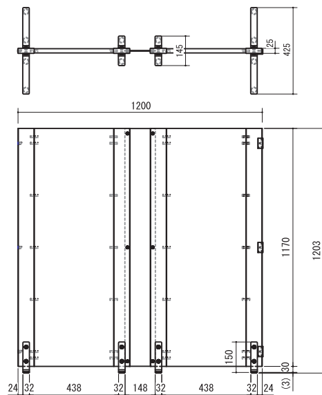
2台連結時
