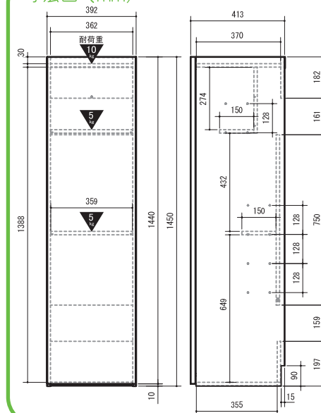
寸法図 (mm)
